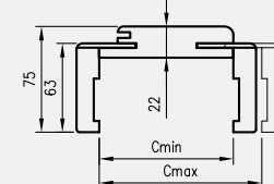
Przekrój OR/ORC z kąt. T63
