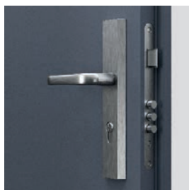
Drzwi Steel SAFE Typ II Zamek dolny – 3 ryglowany
